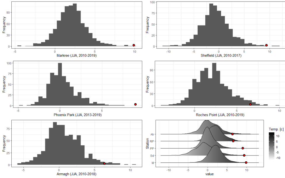
Tmax (°C) JJA Frequency Distribution 2010-2019
