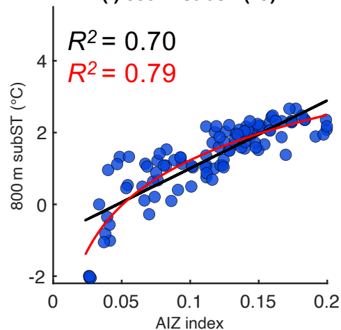
(f) 800 m subST (°C)
