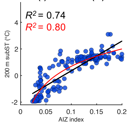
(c) 200 m subST (°C)
