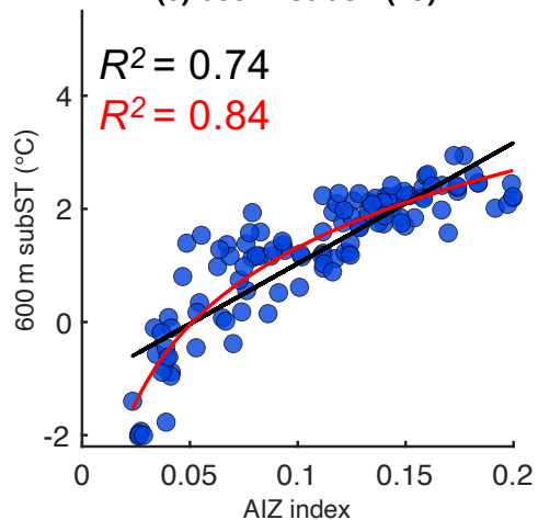
(e) 600 m subST (°C)
