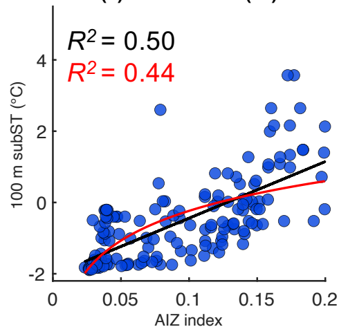
(b) 100 m subST (°C)
