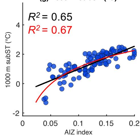
(g) 1000 m subST (°C)
