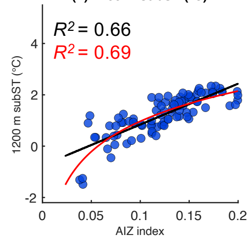
(h) 1200 m subST (°C)
