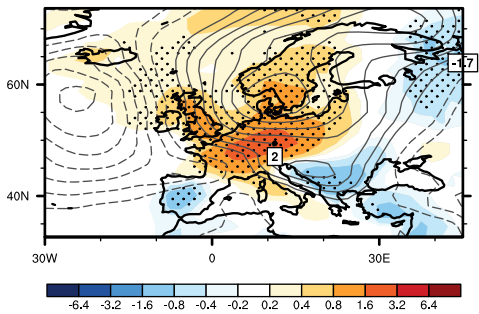
ModE-RA
