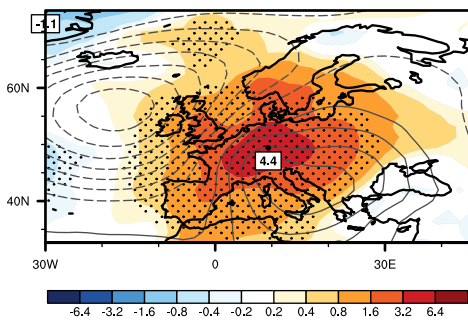
ModE-RA
