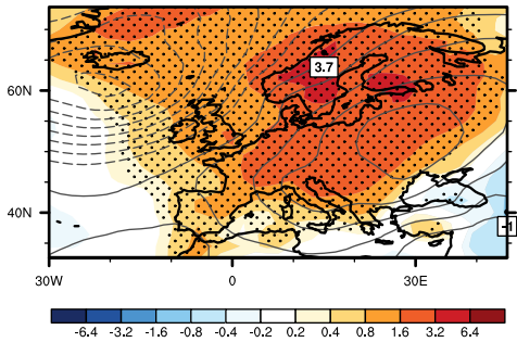
ModE-RA
