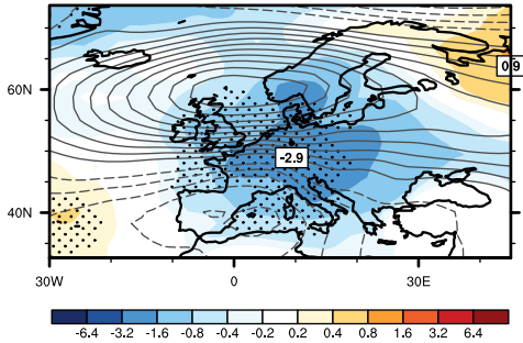
ModE-RA
