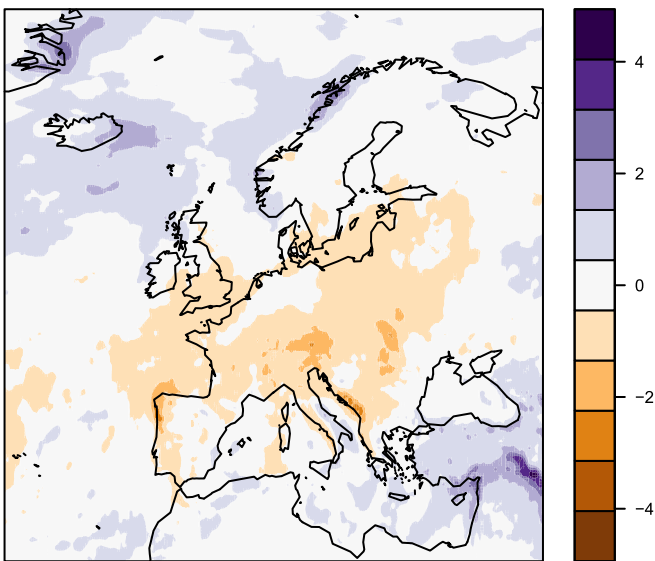
MAM precipitation anomaly (mm/d)
