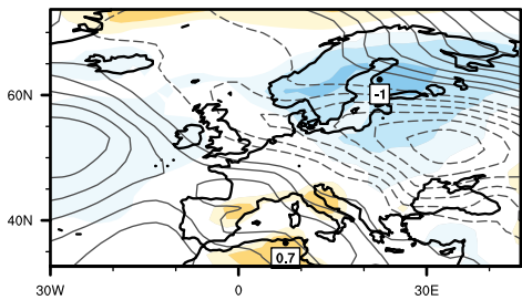
ModE-RA
