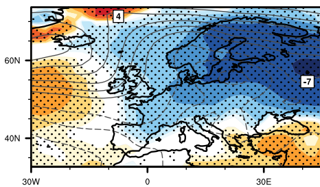
ModE-RA
