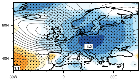
ModE-RA
