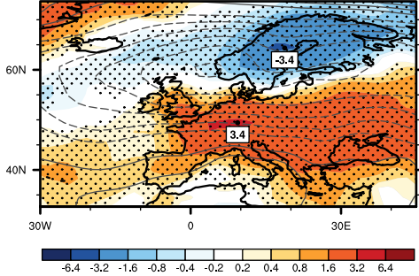
ModE-RA
