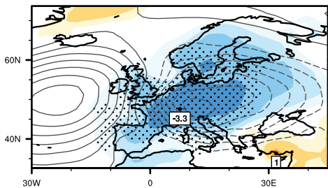
ModE-RA
