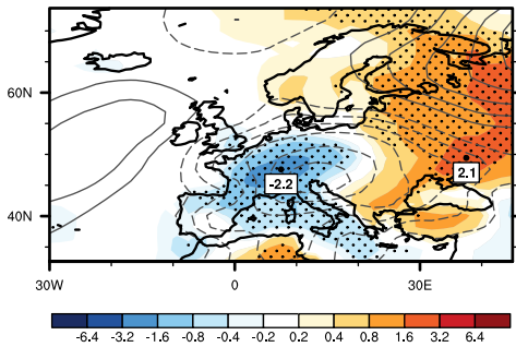
ModE-RA
