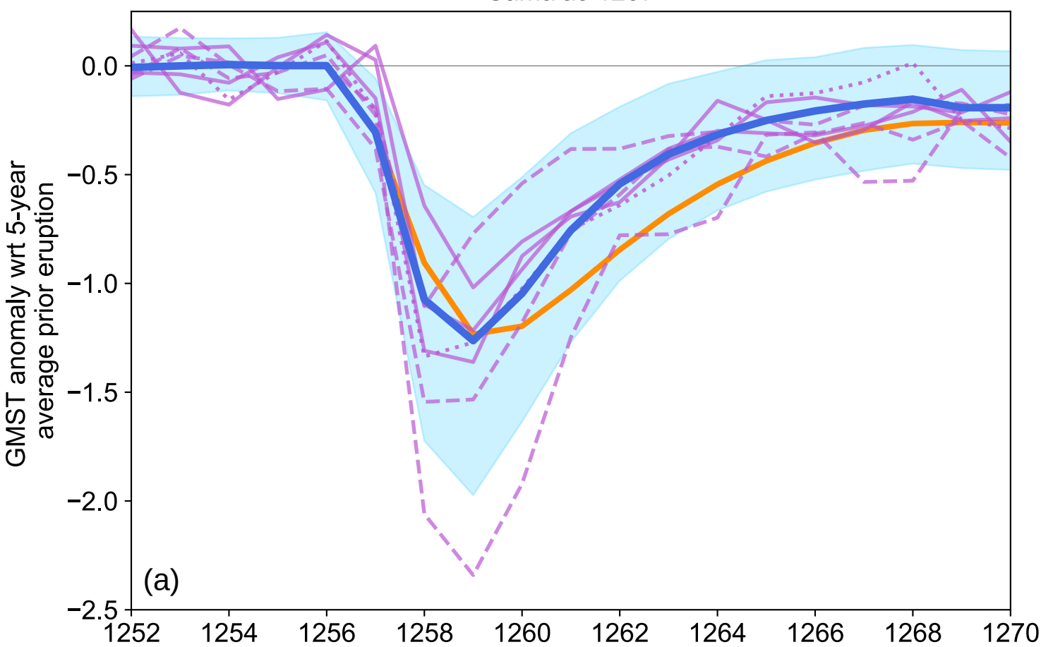
Samalas 1257
