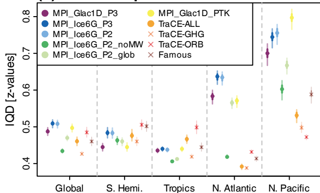
(d) Millennial pattern deviations
