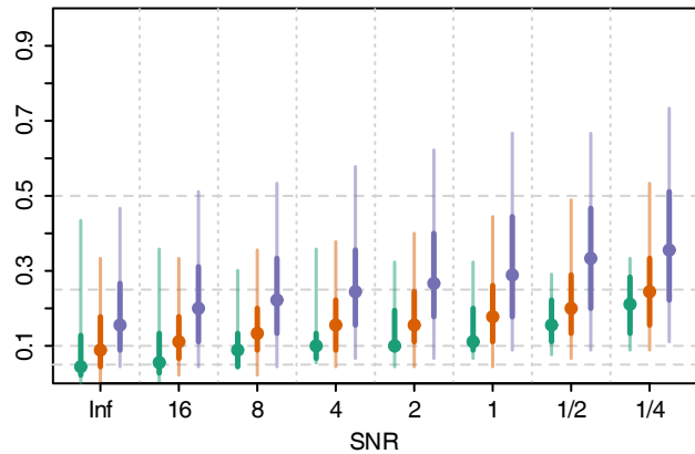
(d) Millennial pattern
