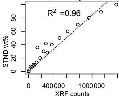
SiO 2
