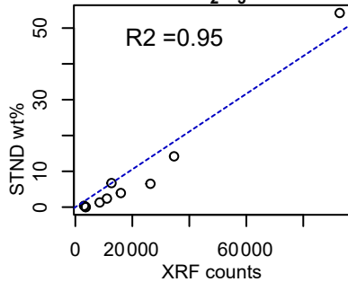
Al 2 O 3
