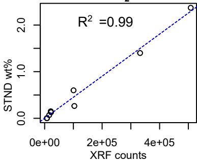
TiO 2
