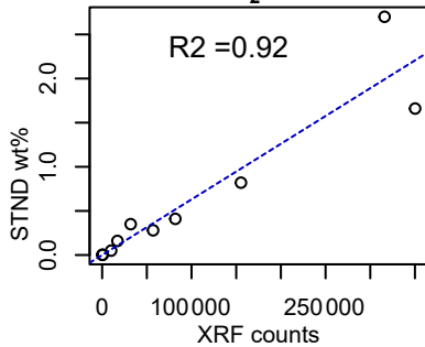
K 2 O
