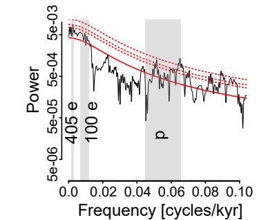
(d) AR1 Confidence Level Estimates
