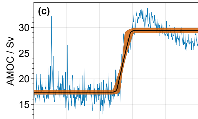
CCSM4 AMOC
