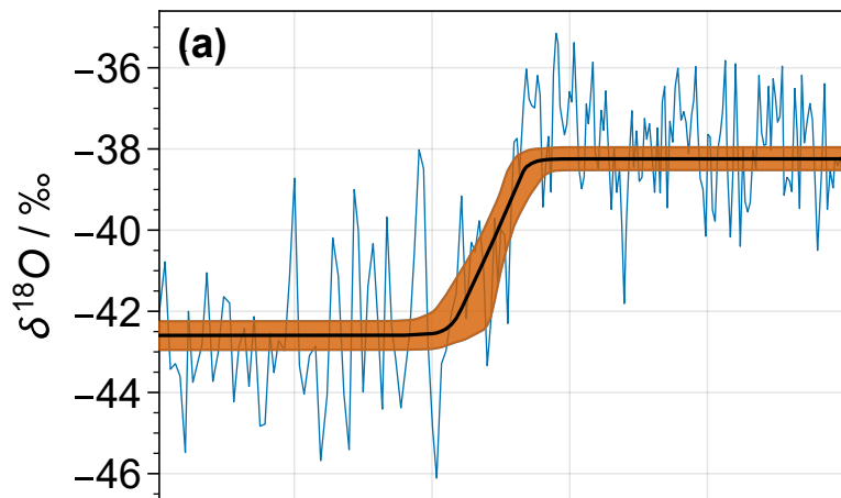
NGRIP \delta^{18}\text{O}
