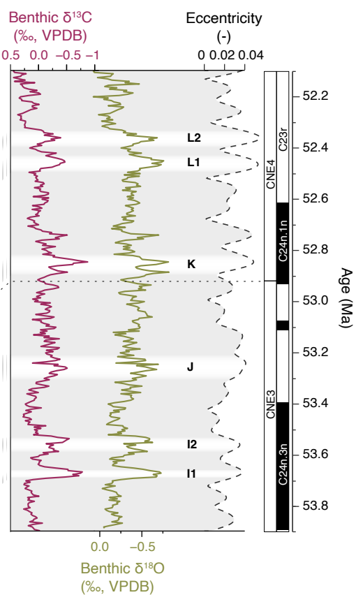
(b) CENOGRID
