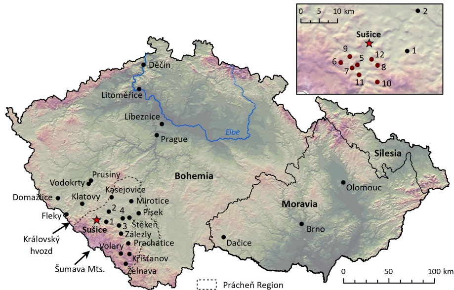
Figure 2. Location of the town of Sušice and other places in the Czech Republic mentioned in the text. The key is as follows: 1 – Bukovník; 2 – Horažďovice; 3 – Nihošovice; 4 – Strakonice; 5 – Dolejší Krušec; 6 – Dolejší Těšov; 7 – Hořejší Krušec; 8 – Humpolec; 9 – Jiříčná; 10 – Kašperské Hory; 11 – Palvínov; 12 – Platoň.
