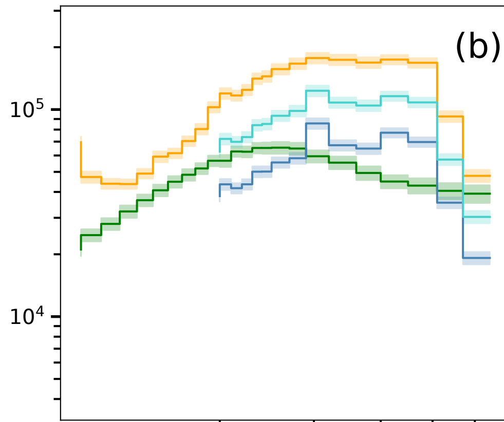
LGM PSD
