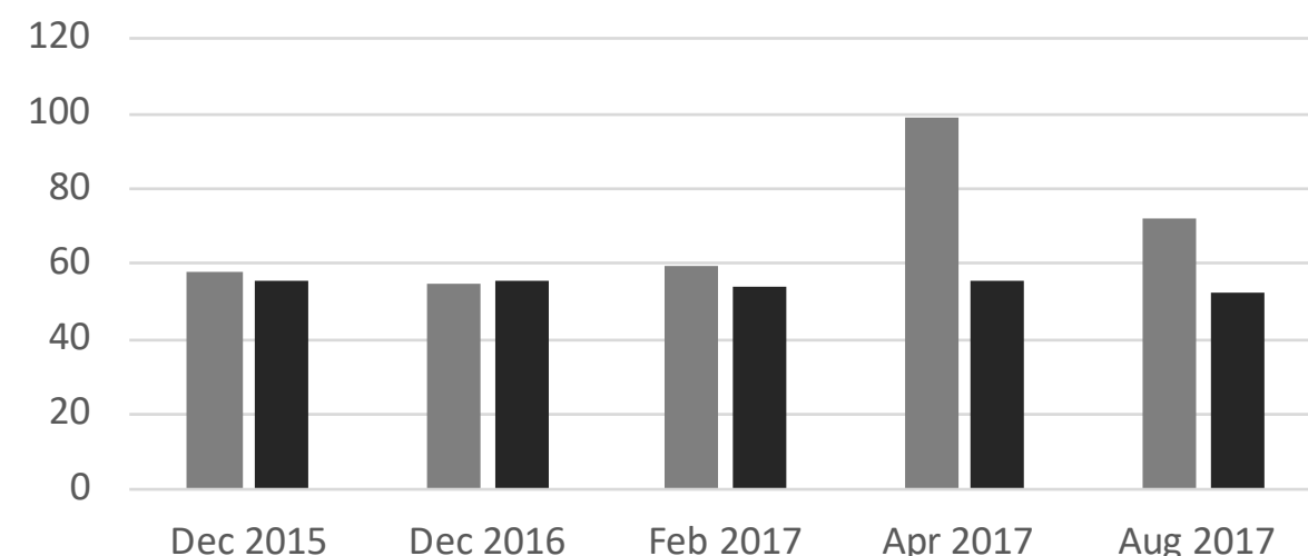
Ti/Zr
