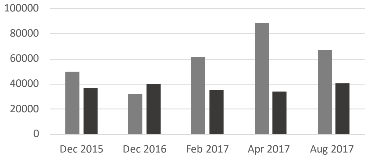
Al ppm
