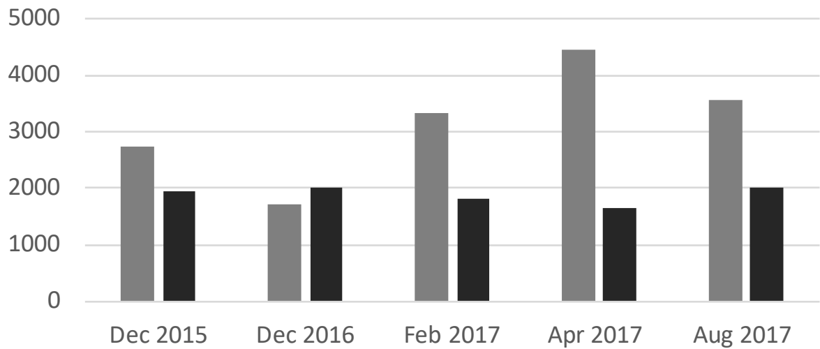
Ti ppm
