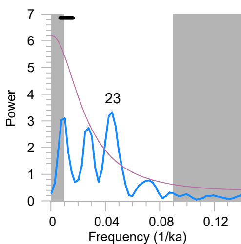
Ericaceae
