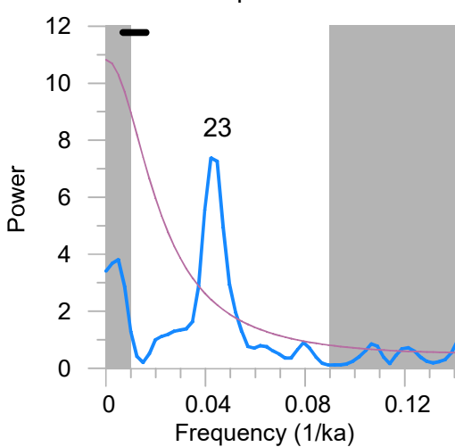
Podocarpaceae
