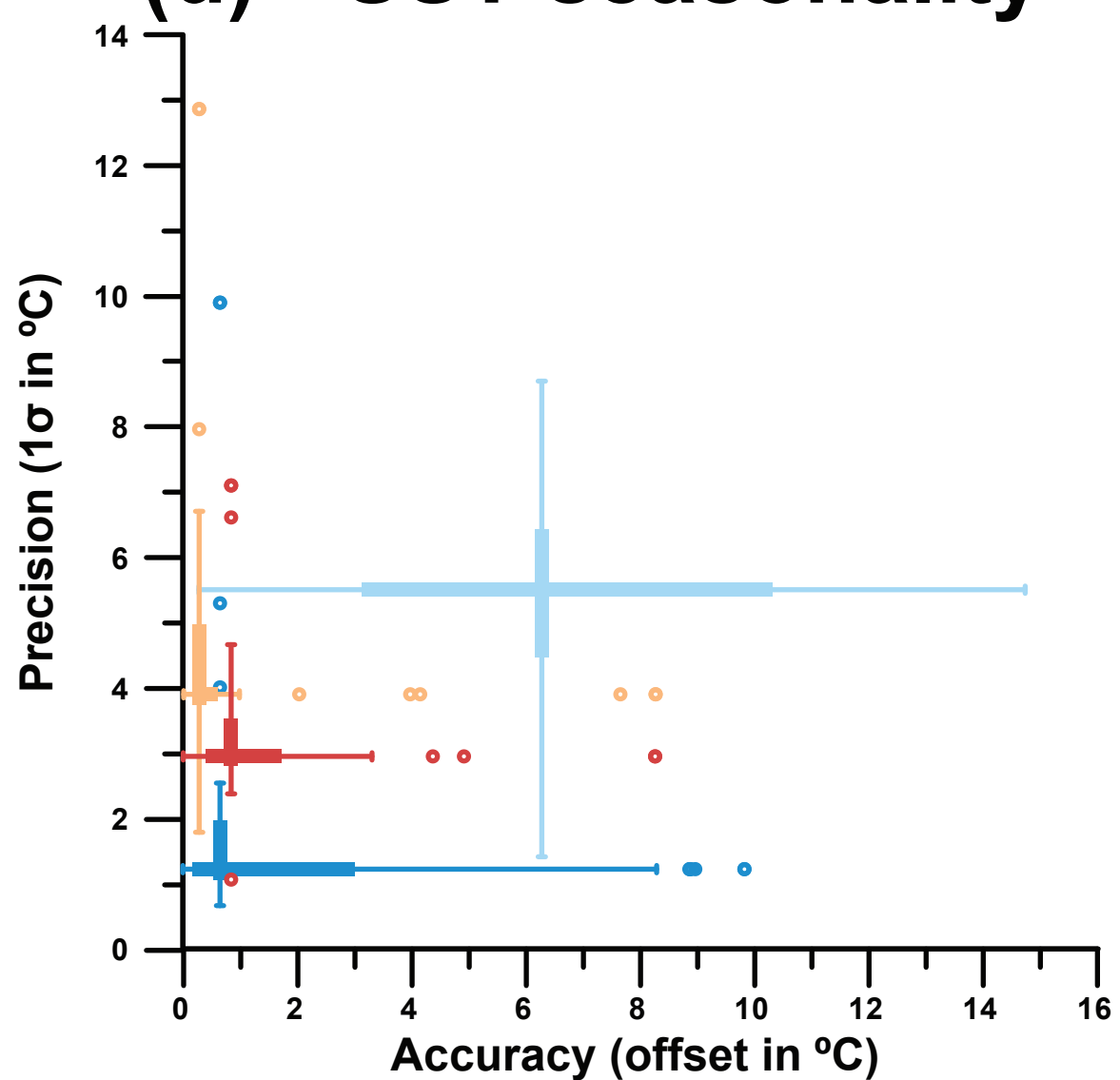
(d) SST seasonality
