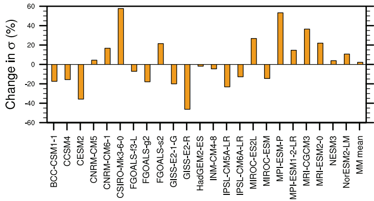
(e) abrupt4xCO2
