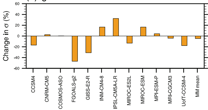
(b) Igm
