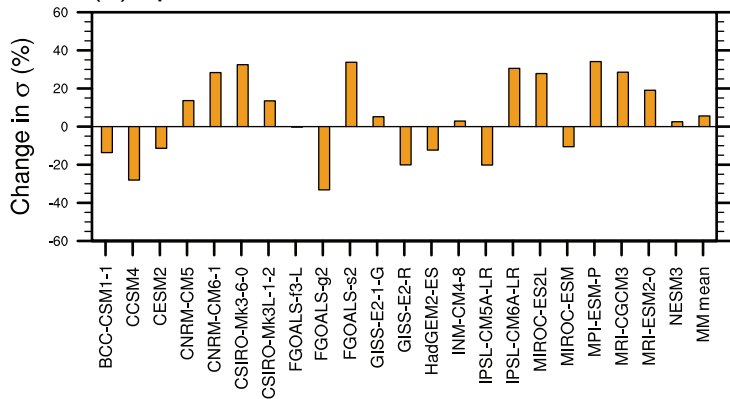
(d) 1pctCO2
