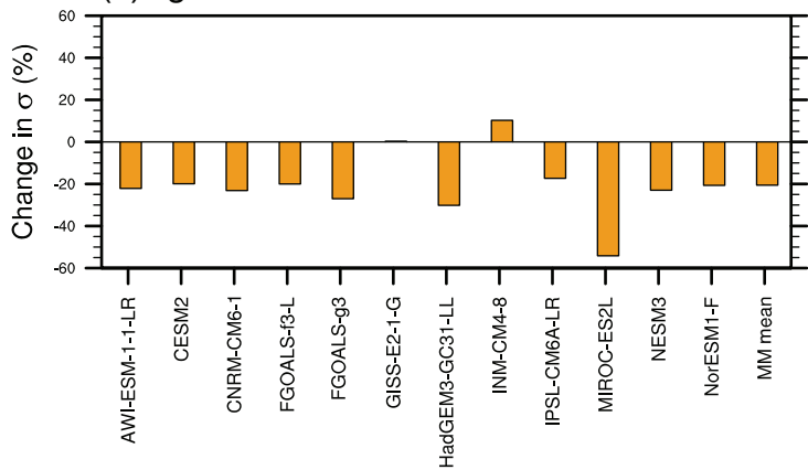
(e) abrupt4xCO2
