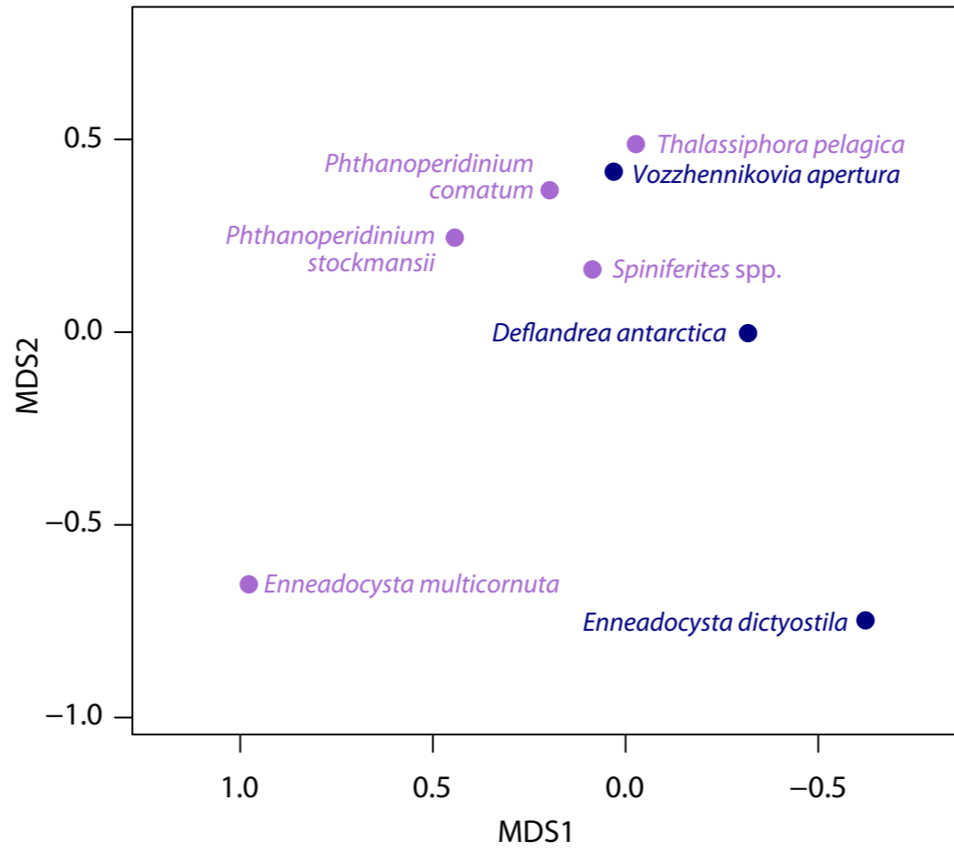
(b) NMDS Site 1172
