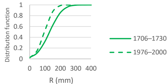
(d) 1706–1730 vs. 1976–2000, spring
