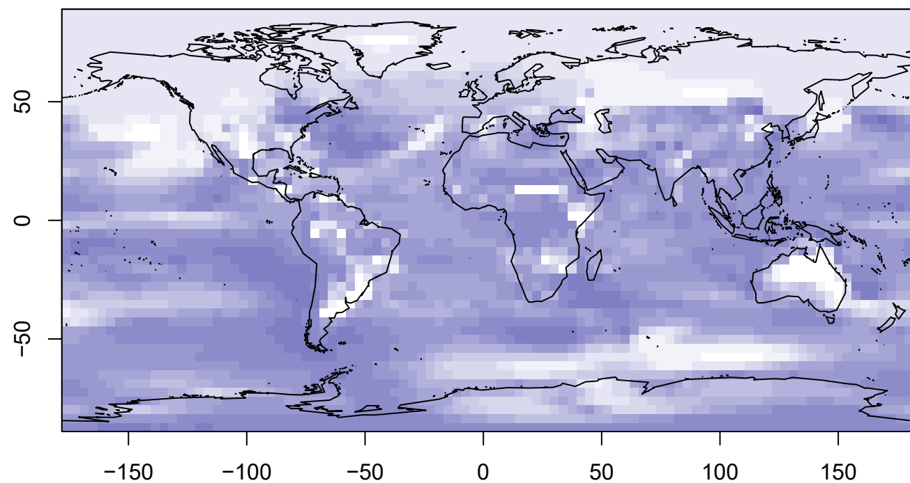
(e) MPI6k
