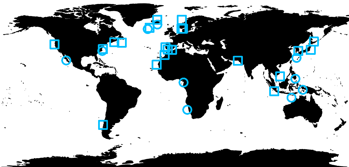
(b) LH14
