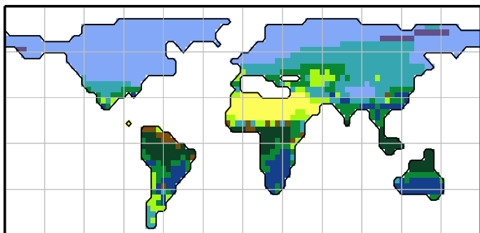
MIROC-ESM
