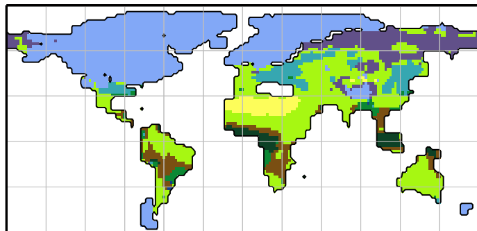
MPI-ESM-T31
