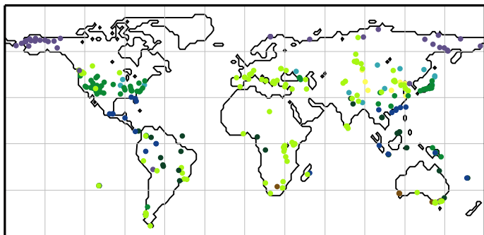
MPI-ESM-T63
