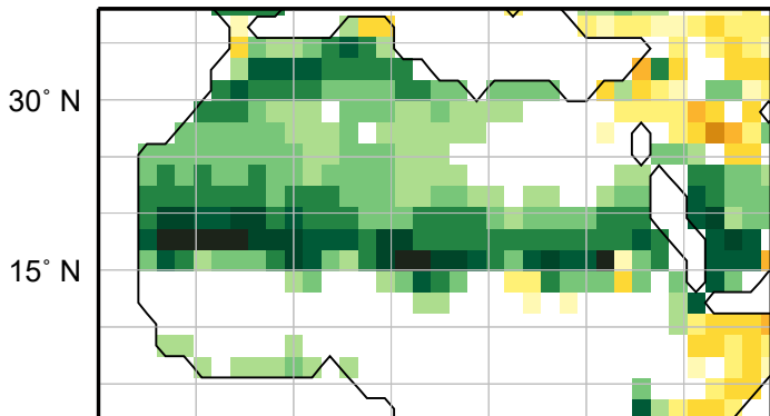
MPI-ESM-T63
