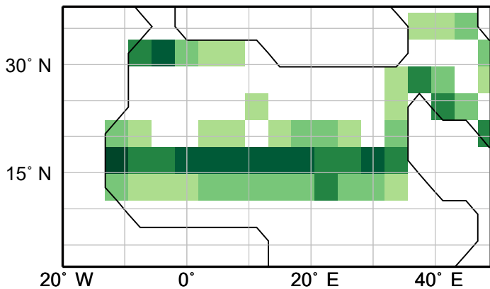
MIROC-ESM
