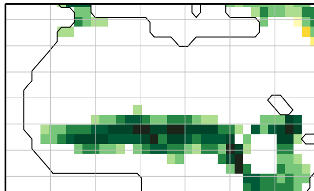
HadGEM2-ESM
