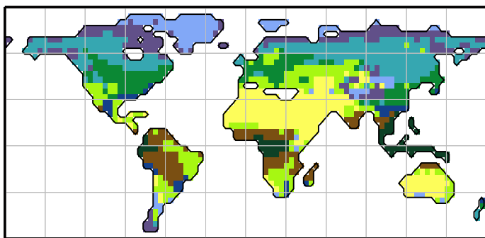
HadGem2-ESM
