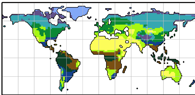
MIROC-ESM
