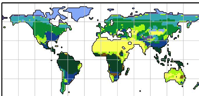
MIROC-ESM
