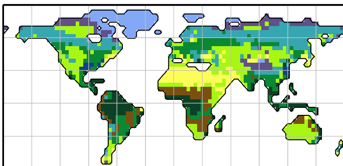
HadGem2-ESM
