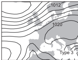
W over S. Europe, cyclonic
