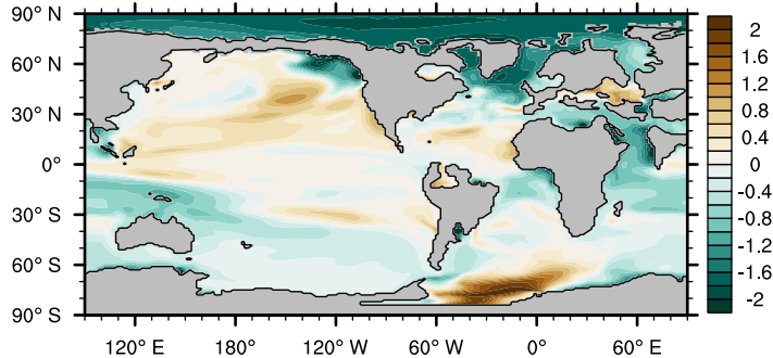
(d) Evap - precip 800 — 400 ppm ( 10^{-5} \text{ kg m}^{-2} \text{ s}^{-1} )
