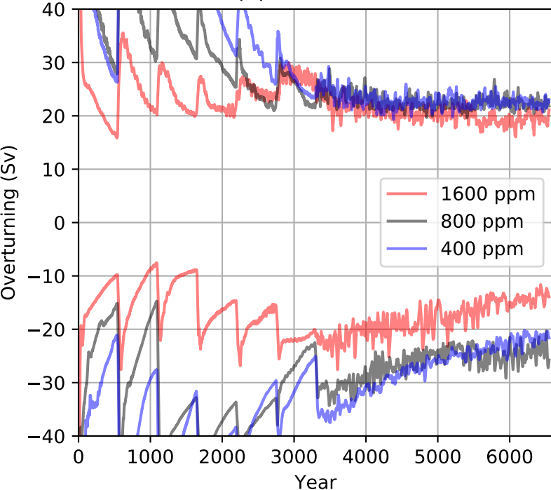
(e) MOC index
