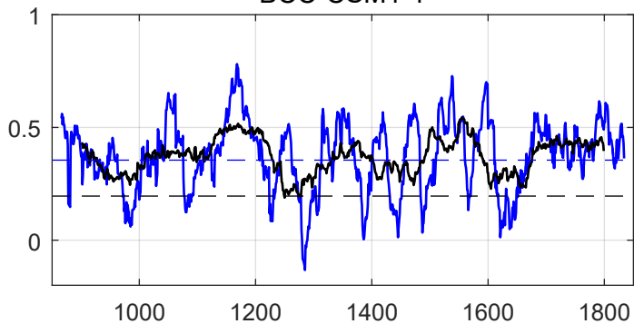
BCC-CSM1-1
