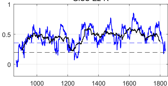
GISS-E2-R
