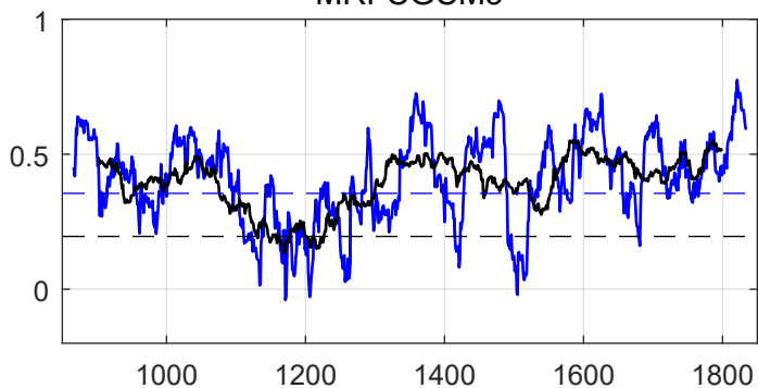
MRI-CGCM3
