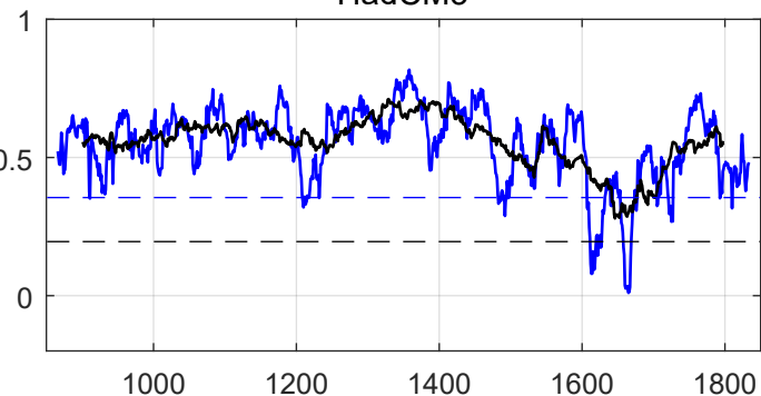
HadCM3
