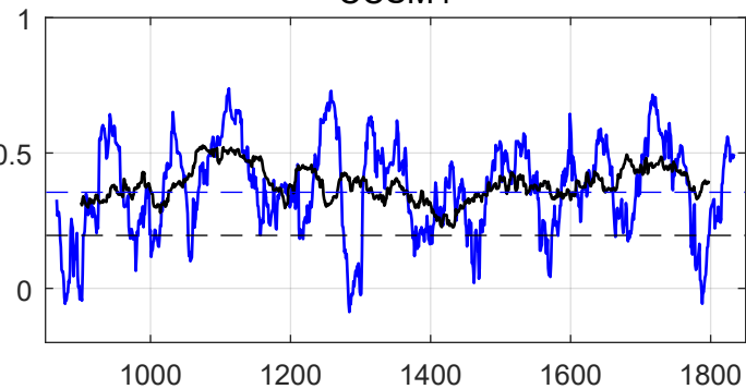
CCSM4
