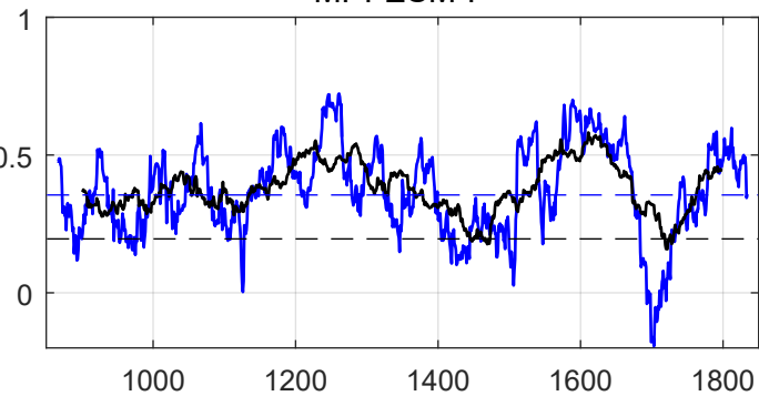
MPI-ESM-P
