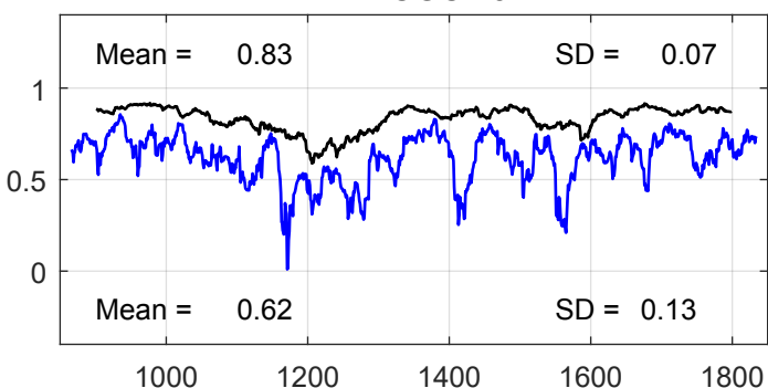
MRI-CGCM3
