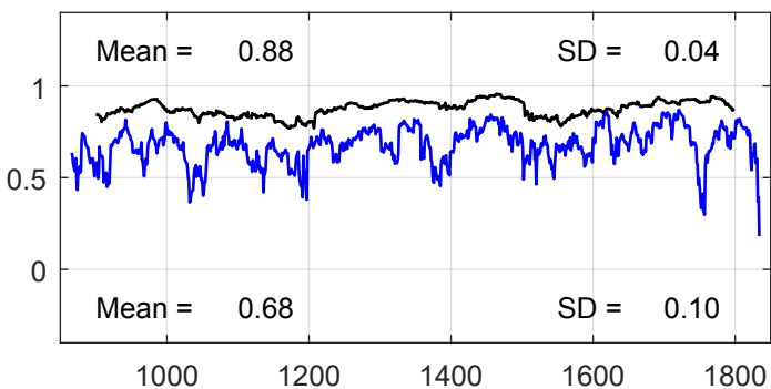
GISS-E2-R
