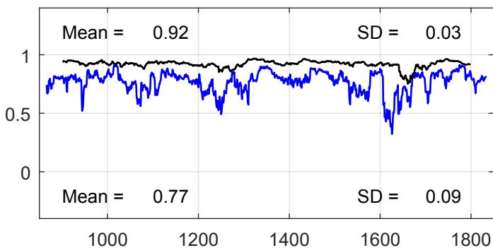
HadCM3
