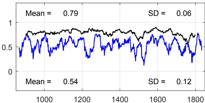
BCC-CSM1-1
