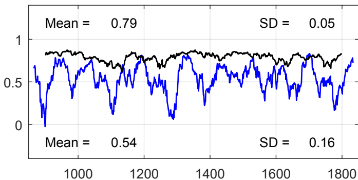
CCSM4
