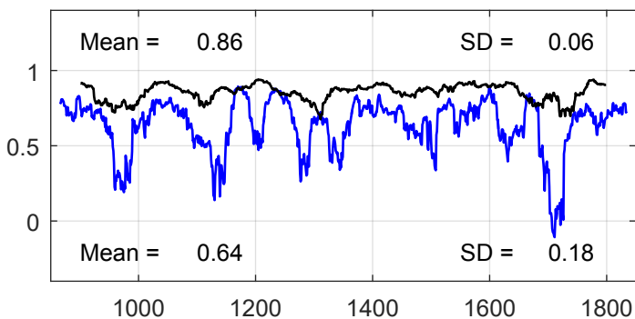
MPI-ESM-P
