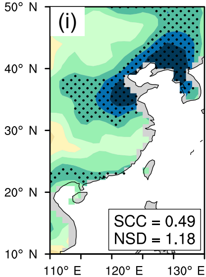
MPI-ESM-P
