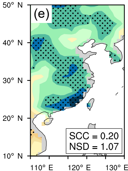
MPI-ESM-P
