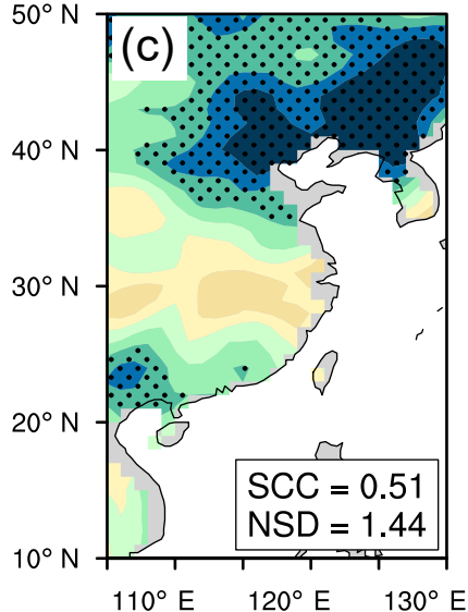
HadCM3
