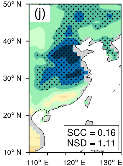
MRI-CGCM3
