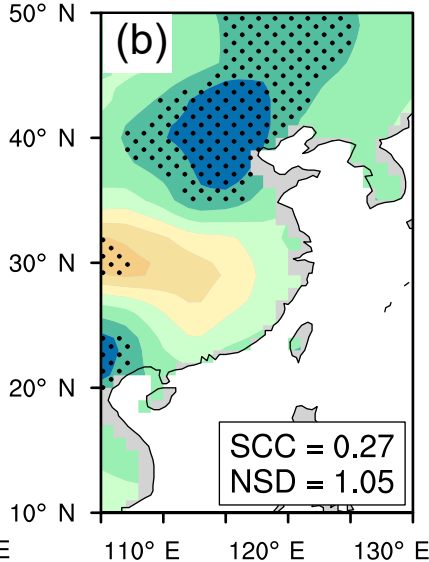
GISS-E2-R
