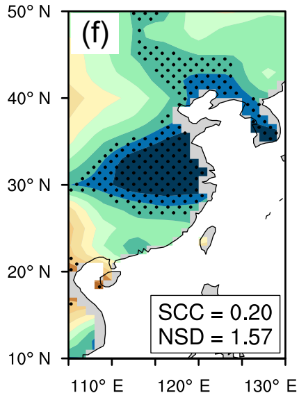
MRI-CGCM3
