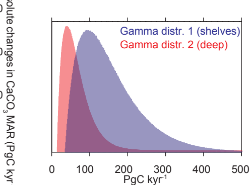
(d) Modern organic carbon burial distribution
