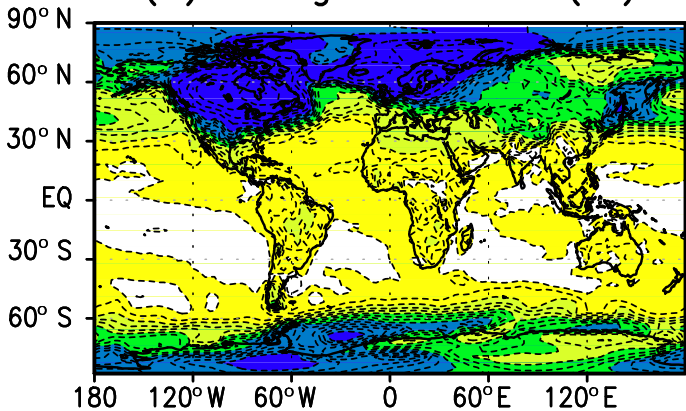
(c) LGMglac.a–LGM.a (°C)
