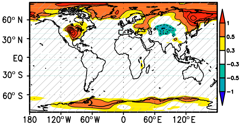
(c) LGMglac.a–LGM.a (°C)
