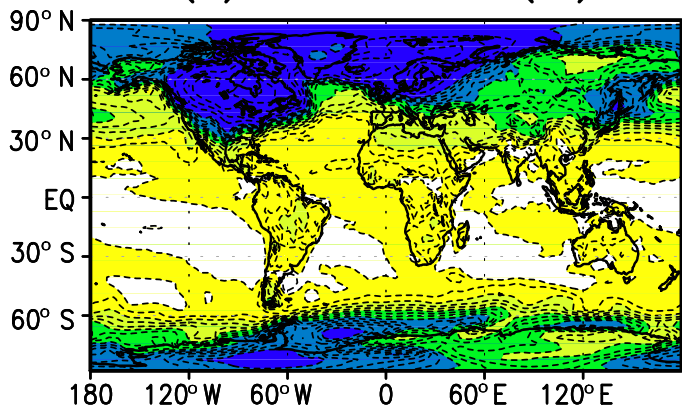
(b) LGMglac.a–Pl.a (°C)
