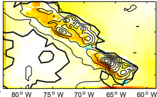
(c) Net CRF (bin It10)– net CRF (bin It1)
