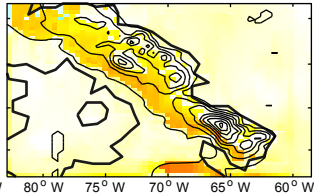
(b) Net CRF (bin It2)– net CRF (bin It1)
