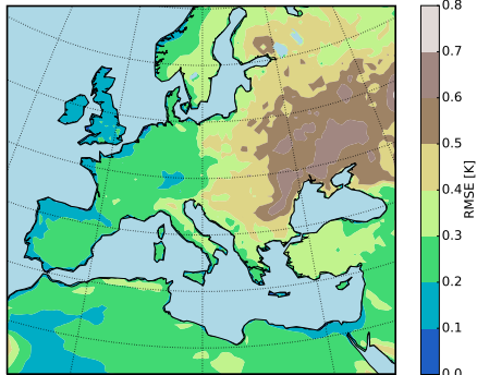
(d) Ensemble RMSE for summer
