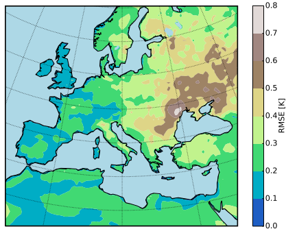
(d) Ensemble RMSE for summer
